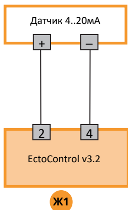
Питание датчика от системы
