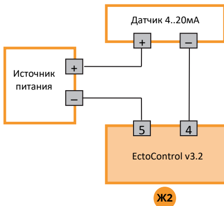
Питание датчика от стороннего источника питания
