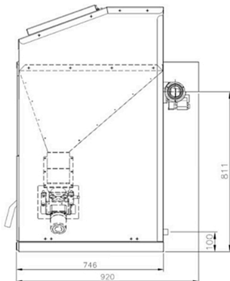
ВИД СБОКУ
